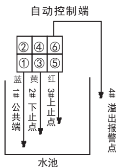
探头联接图
