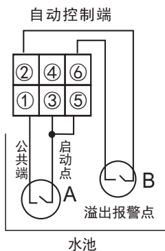
浮球联接图
